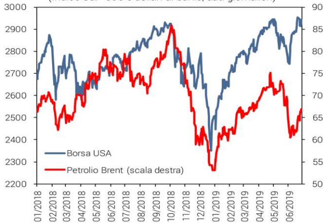
Un ottimo mese per la Borsa USA e il Brent rincarà poco (Indice S&P-500 e dollari al barile, dati giornalieri)
